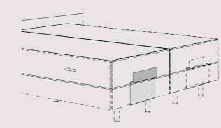
Matratzenbügel für motorisch verstellbare Boxen Mattress support for adjustable motor-driven boxes
