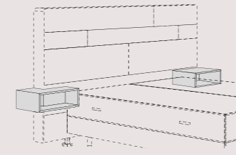
Seitliche Ablagefächer für Stoffkopfteil BC 310 Side storage compartments for fabric headboard BC 310
