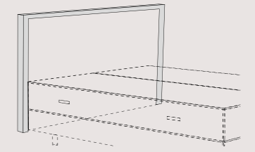
Holzrahmen für BS Kopfteile Wooden frame for BS headboards
